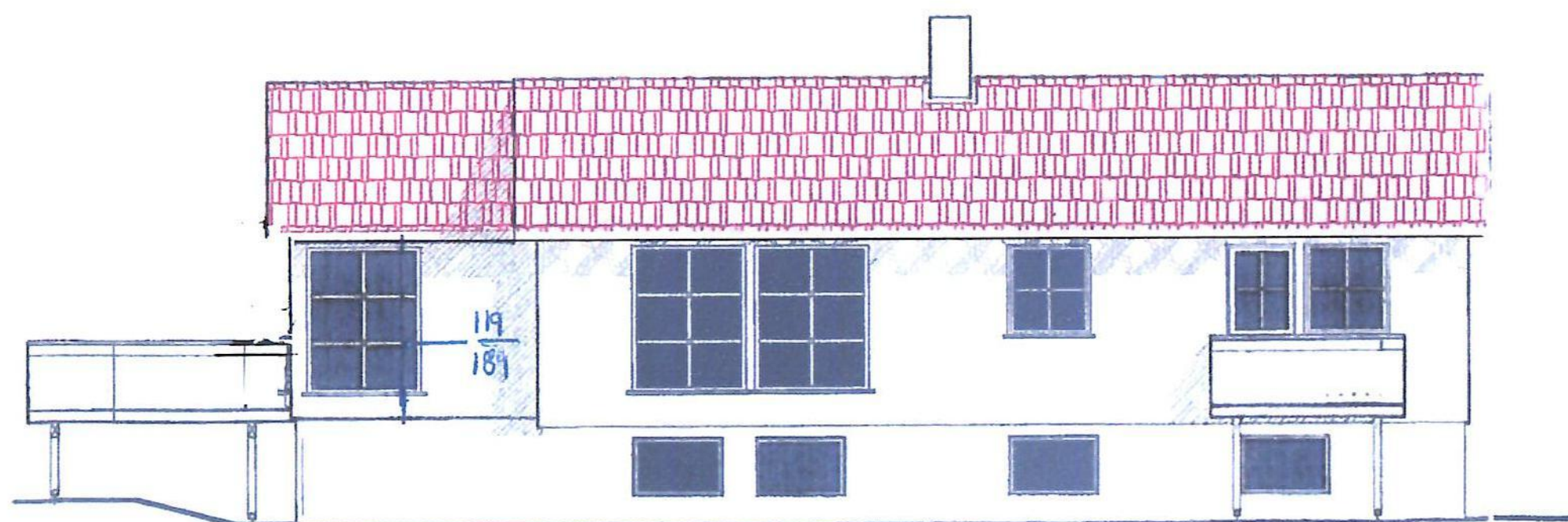
FASADE MOT AUST
