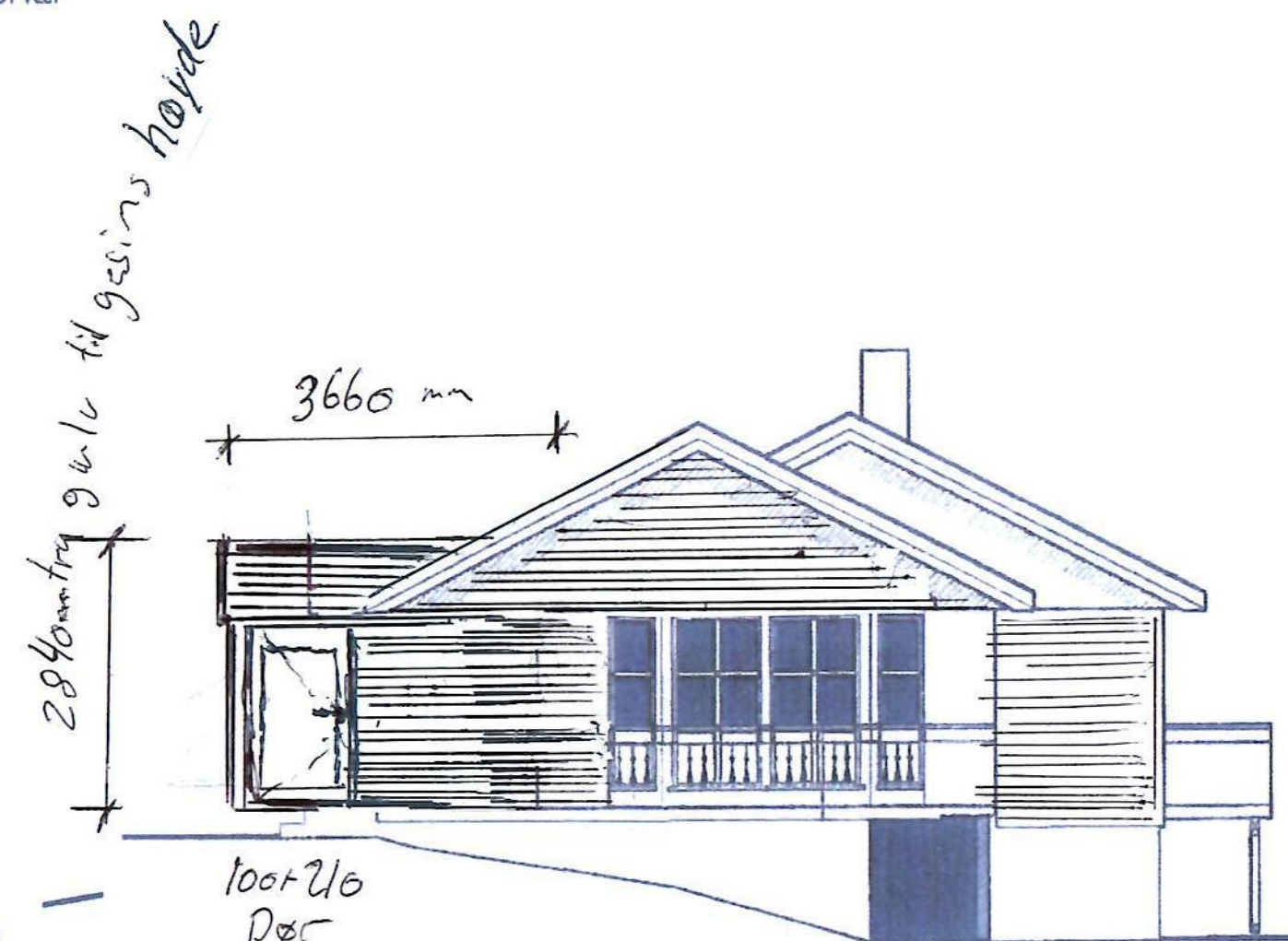
FASADE MOT SØR
